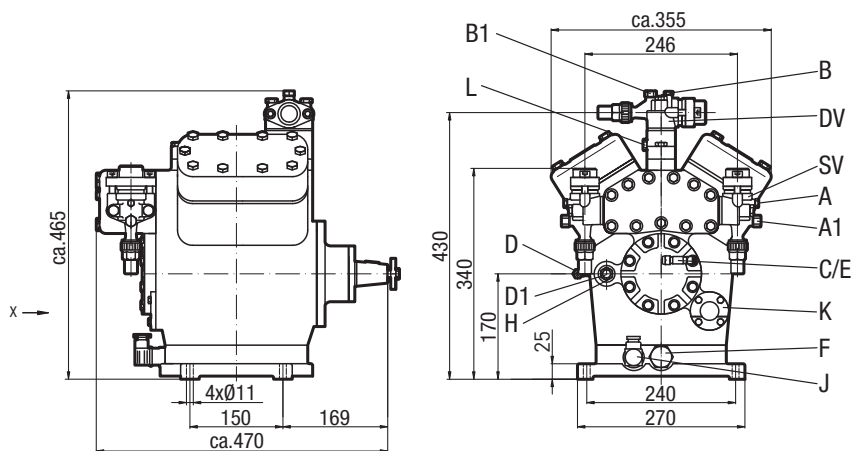
Fig. 26 Dimensions en mm
