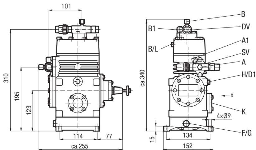
Fig. 20 Dimensions en mm
