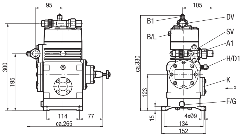
Fig. 33 Dimensions en mm
