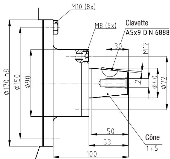
Fig. 27 Dimensions en mm Dimensions pour vue X voir page 31
