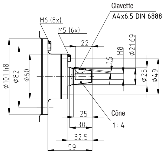
Fig. 34 Dimensions en mm Dimensions pour vue X voir page 39
