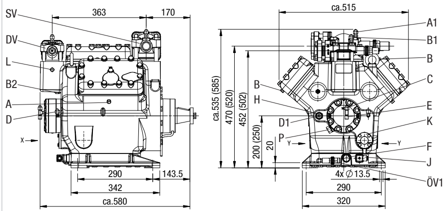
Fig. 30 Dimensions en mm Dimensions en () = Plaque de base élevée
