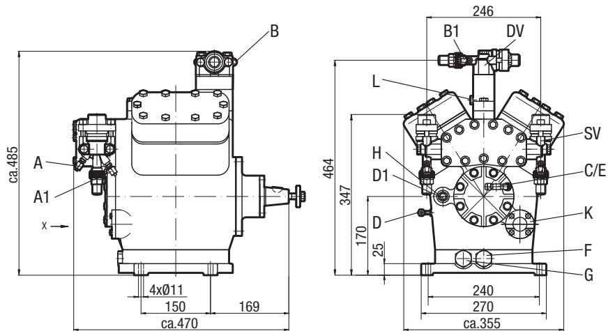
Fig. 39 Dimensions en mm
