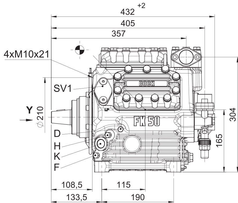
X Ventilausführung K-Version valve version K-version
