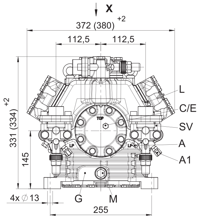
X Ventilausführung N-Version valve version N-version
