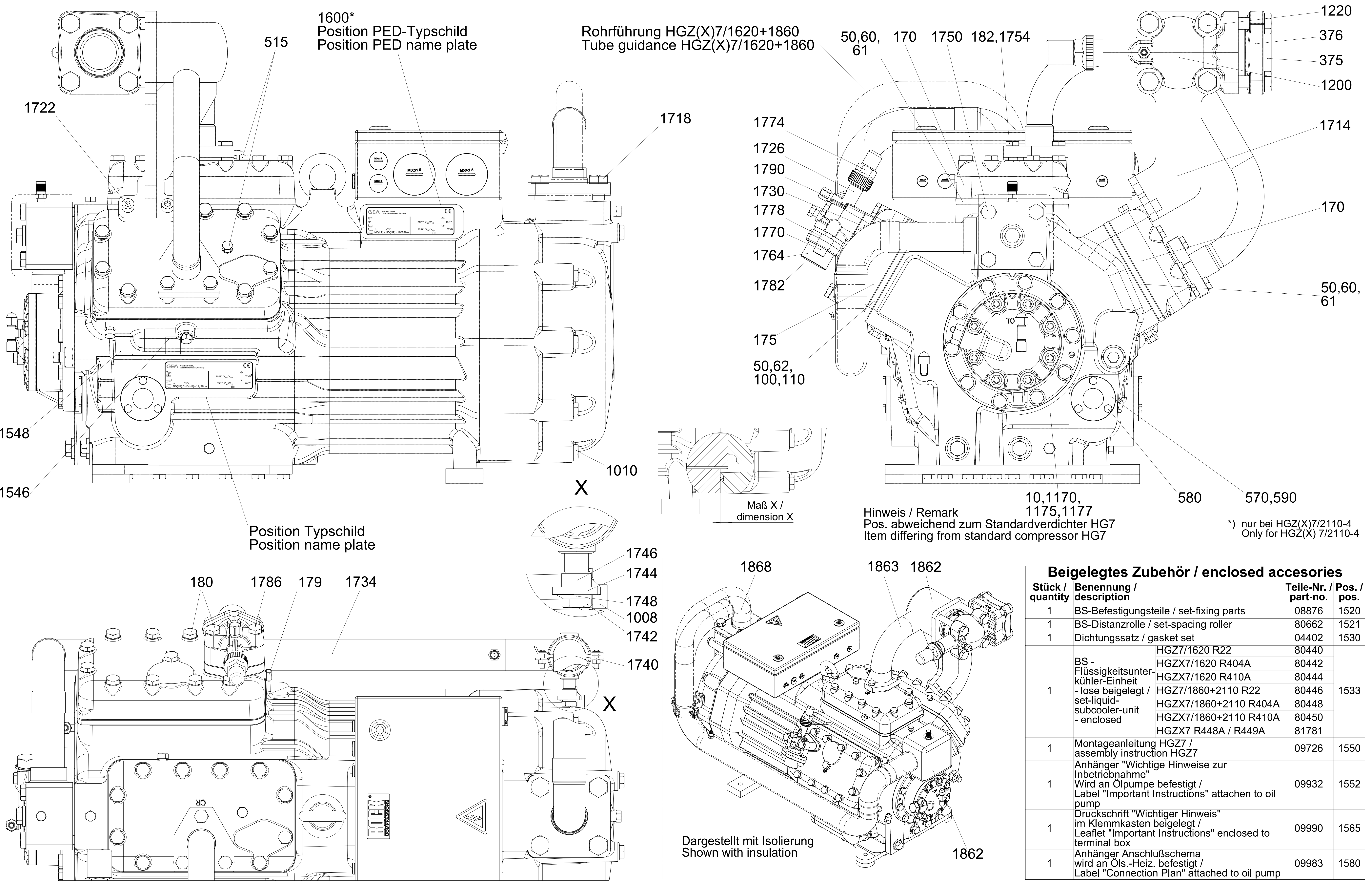
Halbhermetischer zweistufiger Verdichter / Semi-hermetic two-stage compressor
