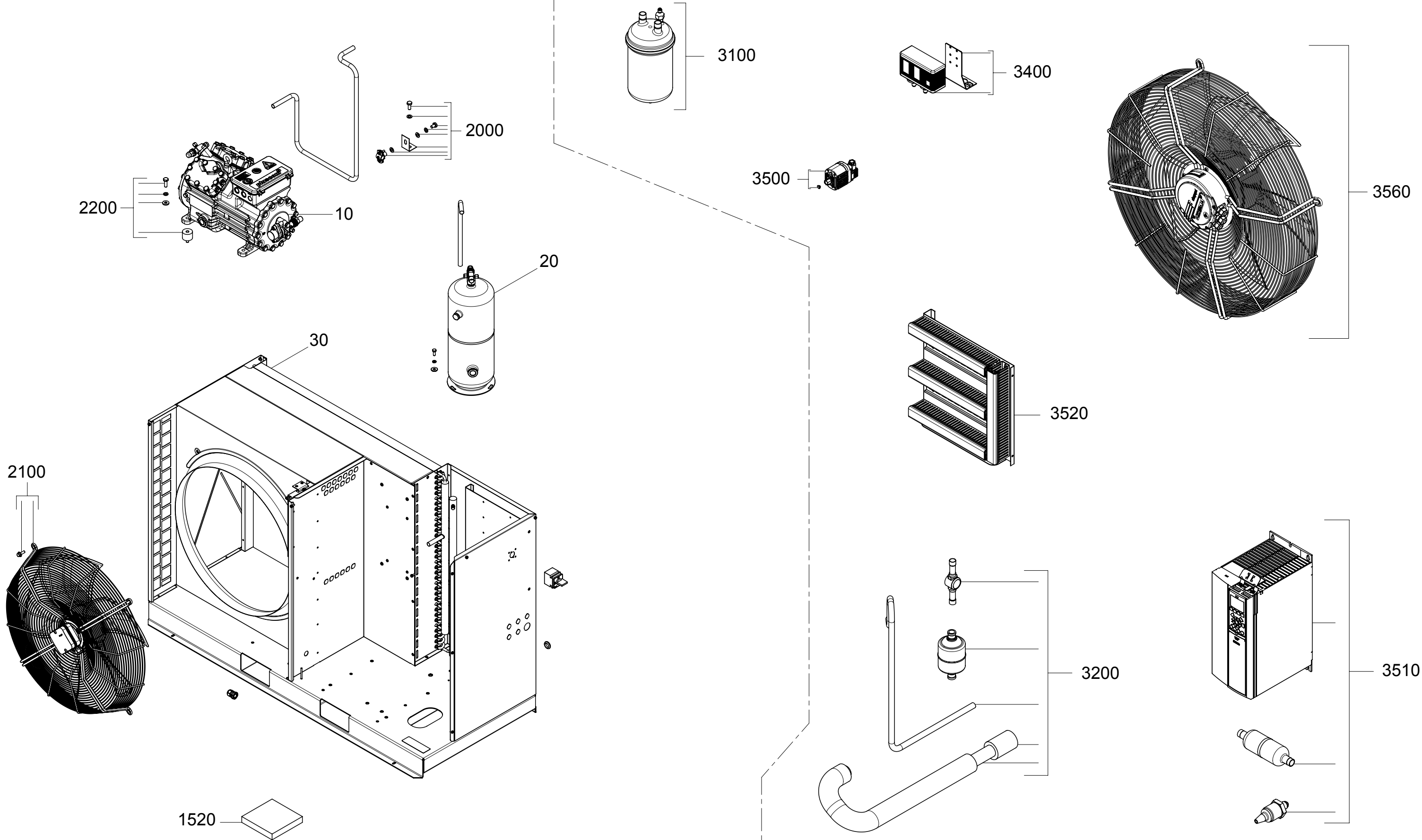
Luftgekühlter Verflüssigungssatz / Air-cooled condensing unit
