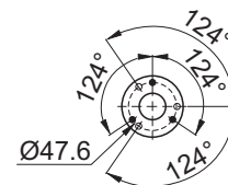
Ansicht X: Anschlussmöglichkeit für Ölspiegelregulator View X: Possibility of connection of oil level regulator
