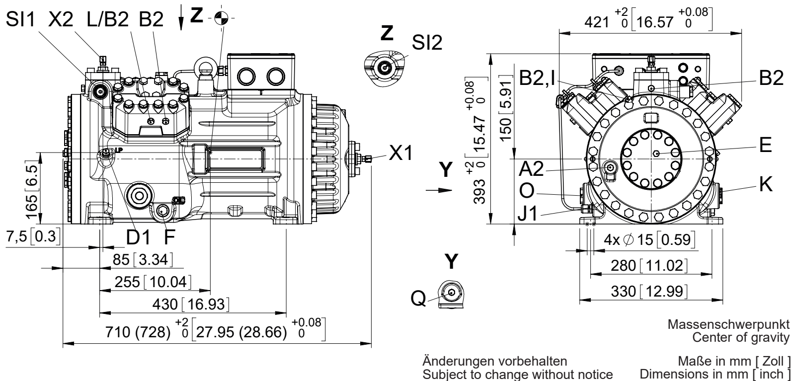
Maße und Anschlüsse mit Absperrventilen Dimensions and connections with shut-off valves
