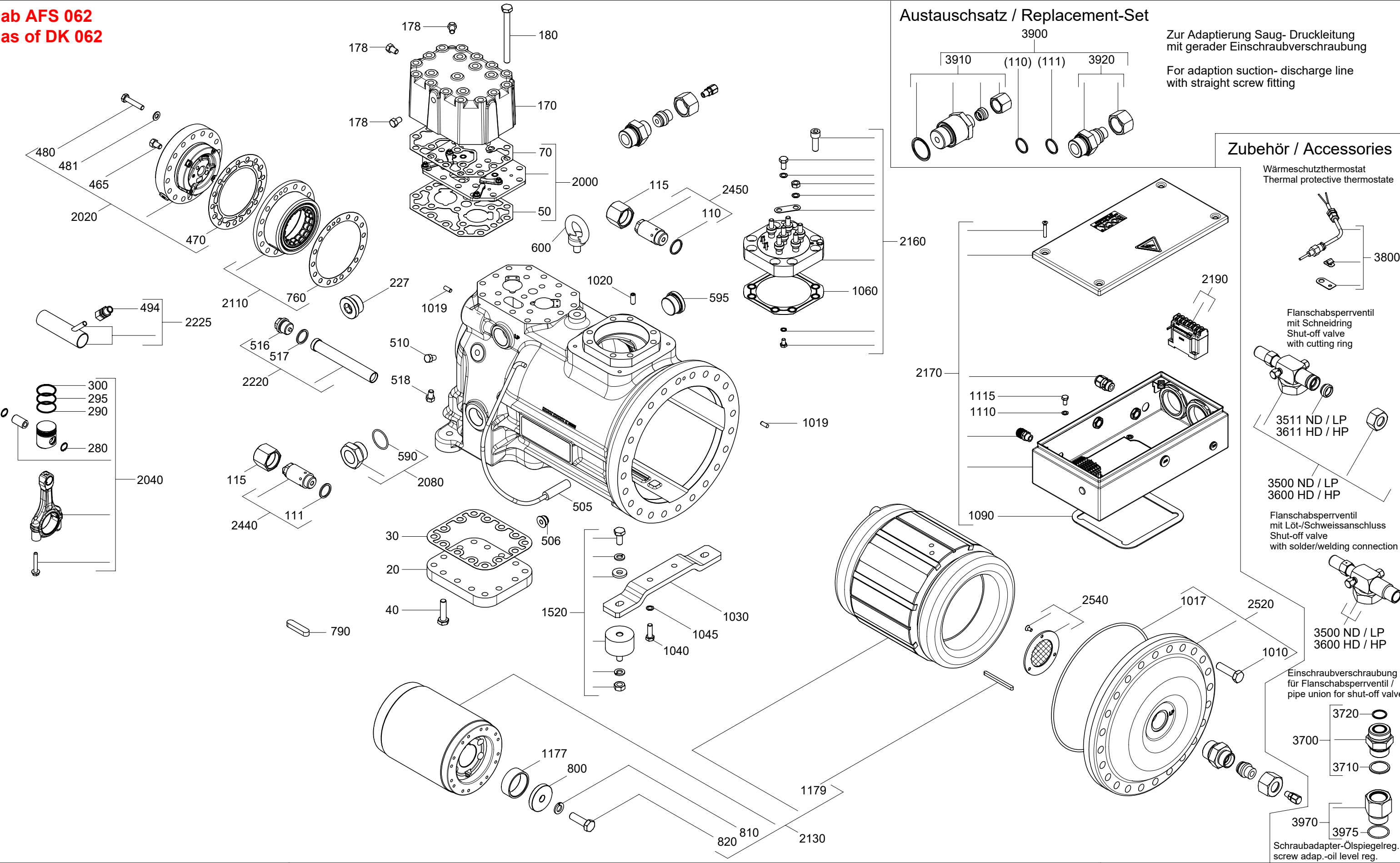
Halbhermetischer Verdichter HG / Semi-hermetic compressor HG
