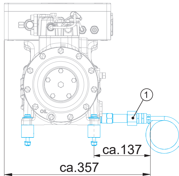
Schwingungsdämpfer Anti-vibration pads
