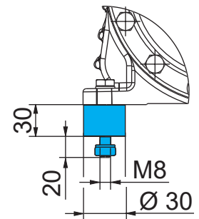
Schwingungsdämpfer Anti-vibration pads
