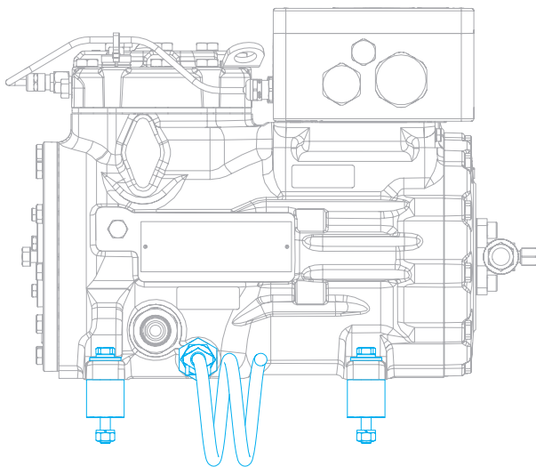
① Ölsumpfheizung / Oil sump heater
