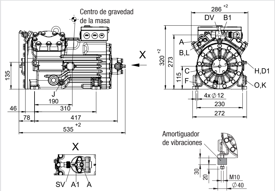
Medidas en mm Fig. 16 1) SV orientable 90° 2) Aprox. 310 mm con caja de bornes en altura de construcción reducida (accesorios)
