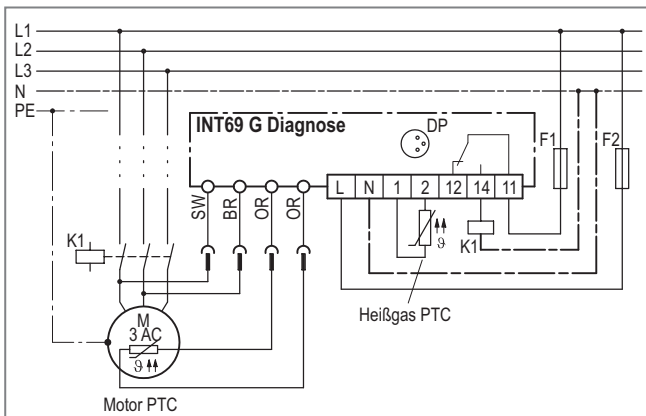
Anschluss-Schaltbild
