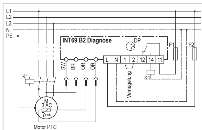
Anschluss-Schaltbild
