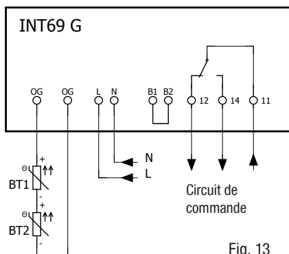
Fig. 13 Boîte à bornes
