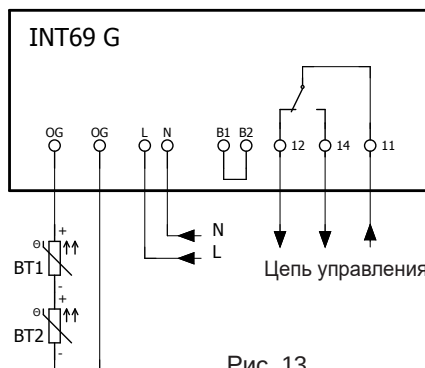
Рис. 13 Клеммная коробка
