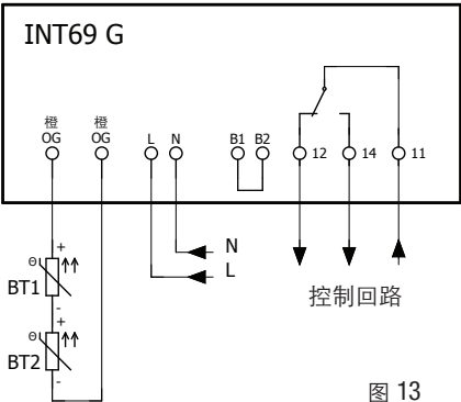
图 13 接线盒
