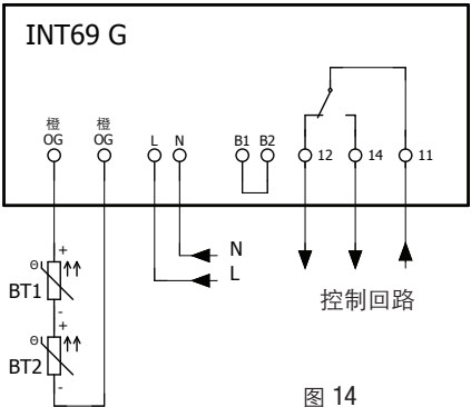
图 14 接线盒
