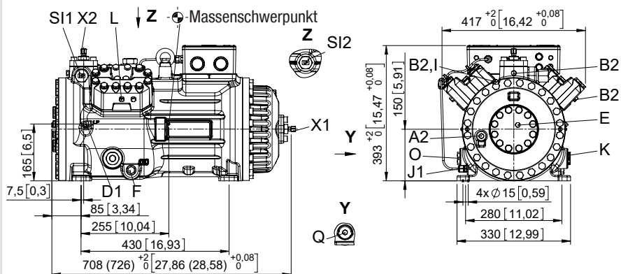
Maße und Anschlüsse mit Absperrventile
